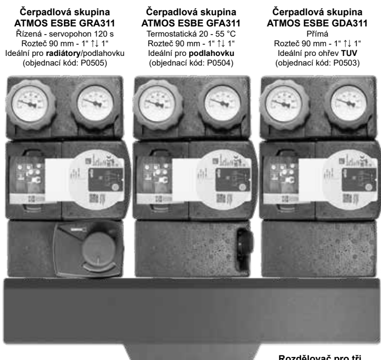
Rozdělovač pro tři čerpadlové skupiny (tříokruhový) ATMOS ESBE GMA331 Rozteč 90 mm - 1" ↑↓ 1" (objednací kód: P0507)
