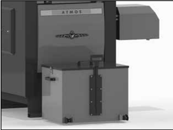
Großer zusätzlicher Aschenkasten für automatische Ascheentleerung (160 l), am Kessel angebracht
