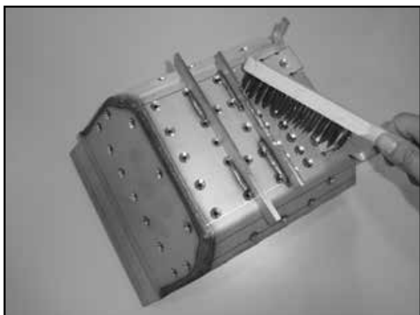
Reinigung der Verbrennungskammer
