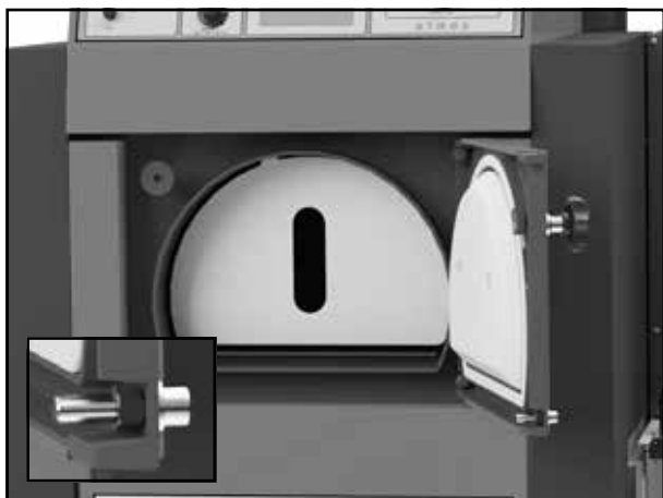
Herausnehmbare, vordere Schutzblende aus Ni-rosta mit Schauloch Sicherungsschraube Tür
