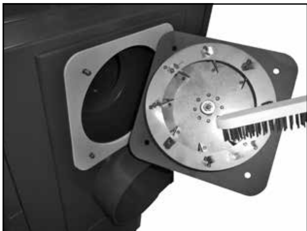
Die Reinigung des Umlaufrad bei Abzugsventilator
