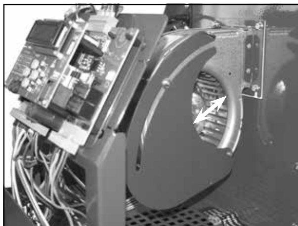
Brennerventilator mit der Luftklappe. Durch Öffnen der Luftklappe wird die Flammenlänge verkürzt.
