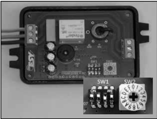
Für die Einstellung geöffnetes Modul AD01 - unter dem Gerätegehäuse des Kessels angebracht
