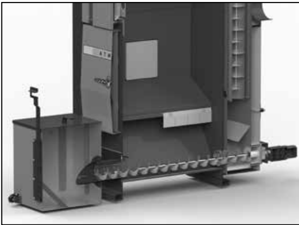
Schnitt: Kessel mit automatischer Ascheentleerung und zusätzlichem Aschenkasten (160 l)
