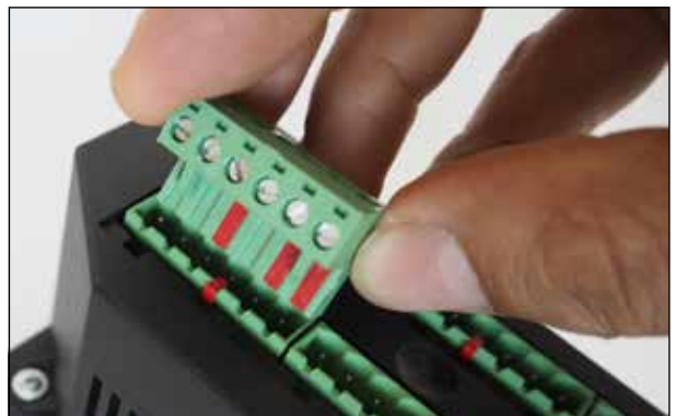
Uwaga – złącza wyposażone są w piny zapobiegające ich zamianie na liście zaciskowej
