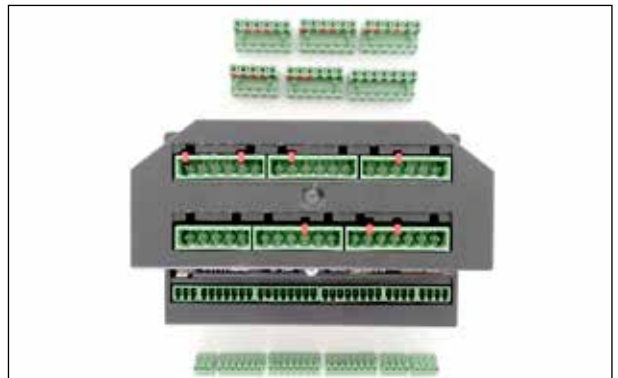
Górne złącza dla elementów wykonawczych Dolne złącza do podłączenia czujników
