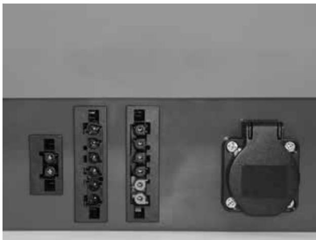
Obr. 12 - hořák - dva 6-pinové konektory, levý sílový, pravý pro čidla, 2-pinový konektor pro přídavný kabel (R3 a R4) a zásuvka pro dopravník
