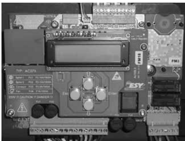
Obr. 5 - elektronická řídicí jednotka s tlačítky, spodní svorkovnice (1 - 18), vrchní svorkovnice pro připojení čidel TS, TV, TK, TSV a fotocely s rozšiřujícím modulem AC07X-C (R5, R6)
