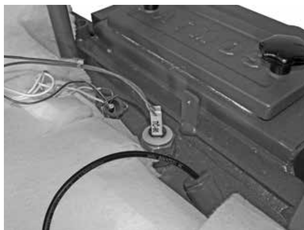
Obr. 16 - pohled na čidlo teploty vody TK v jímce kotle DC40SPT, DC40GSP
