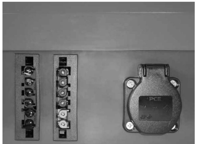
Abb. 12 - Brenner / zwei 6 Pin konektore, links Spannung, rechts Fühler und Steckdose für Förderschnecke
