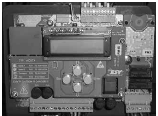
Abb. 6 - Elektronische Steuereinheit mit Tasten, ausgeführt für Kessel PXXx, Pxx Compact, DxxPX, mit zusätzlichem Modul AC07X-C (R5, R6)
