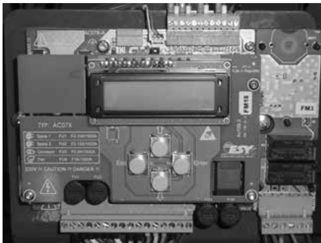
Obr. 6 - elektronická řídicí jednotka s tlačítky v provedení pro kotle DxxPX, PXxx, Pxx Compact s rozšiřujícím modulem AC07X-C (R5, R6)
