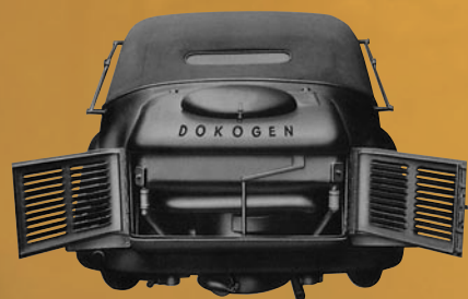
Škoda SUPERB s generátorem DOKOGEN r. 1943
