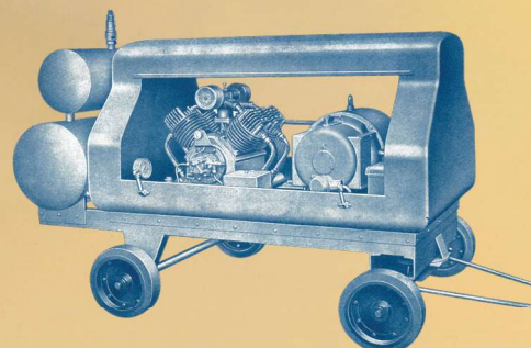
Pojízdná kompresorová souprava ATMOS typ V-4-RZE r. 1950
