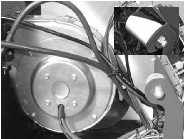
Abb. 9 - Ventilator mit dem Drehzahlgeber und Anlaufkondensator
