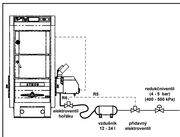
Schaltung mit dem zweiten Elektroventil und einem zusätzlichen Luftspeicher
